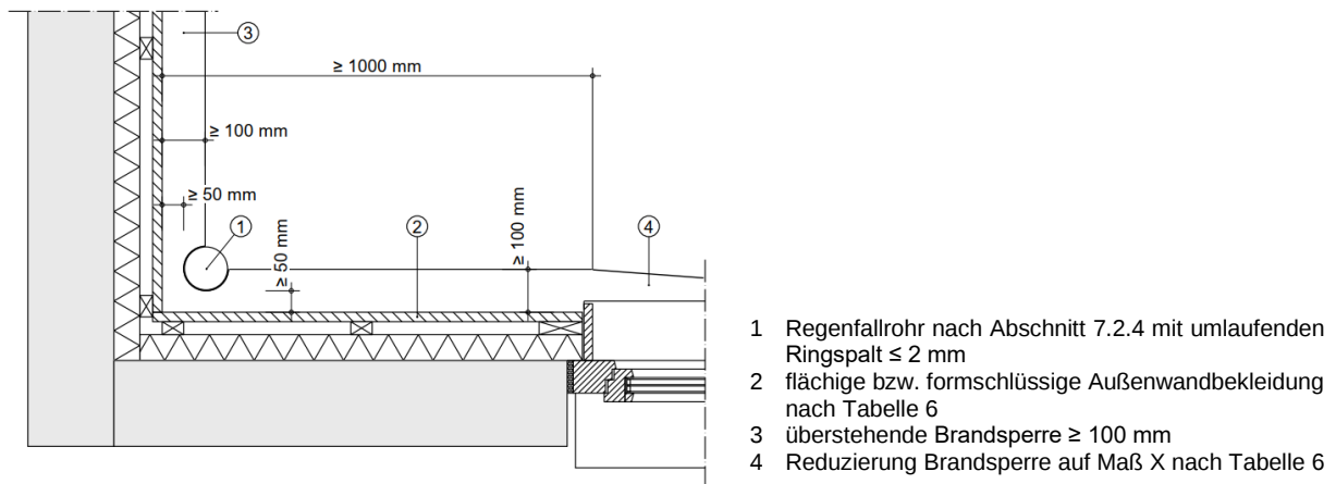
Prinzipiskizze 8: Überstehende horizontale Brandsperre in Innenecke, hier: flächige Holzwerkstoffplatte (Horizontalschnitt)
