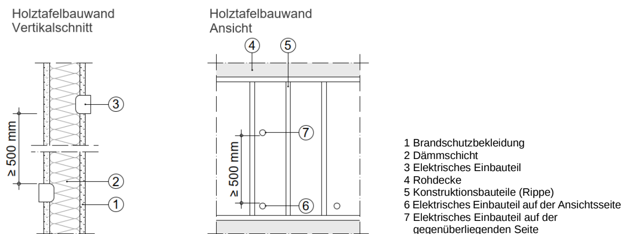
Prinzipiskizze 4: Anordnung von elektrischen Einbauteilen in Holztafelbauwänden
