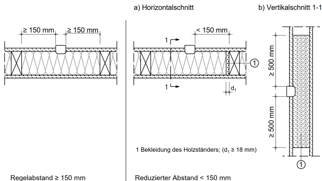
Prinzipische Skizze 5: Regel- und reduzierter Abstand von elektrischen Einbauteilen zu brennbaren Konstruktionsbauteilen
