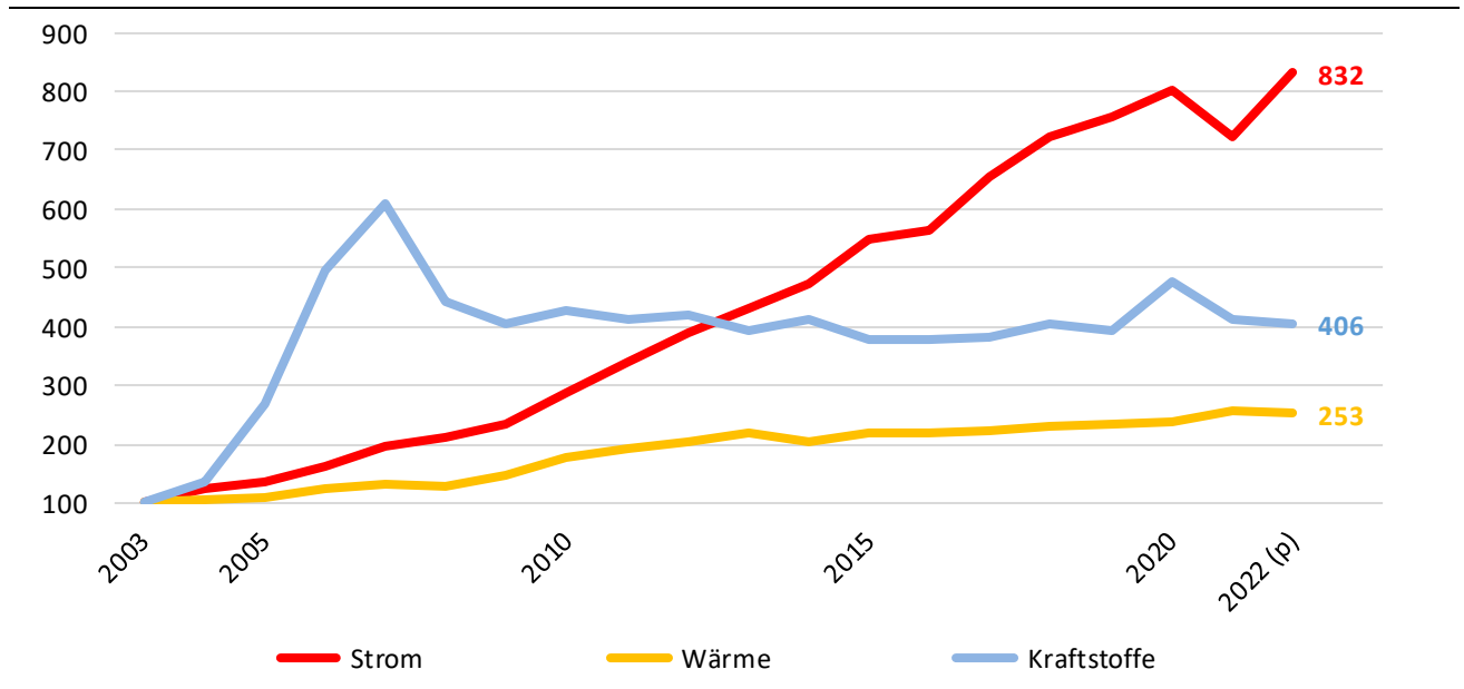
Abbildung 23: Entwicklung des EEV von Strom, Wärme und Kraftstoffen aus erneuerbaren Energien 2003*-2022 (Index 2003 = 100)
