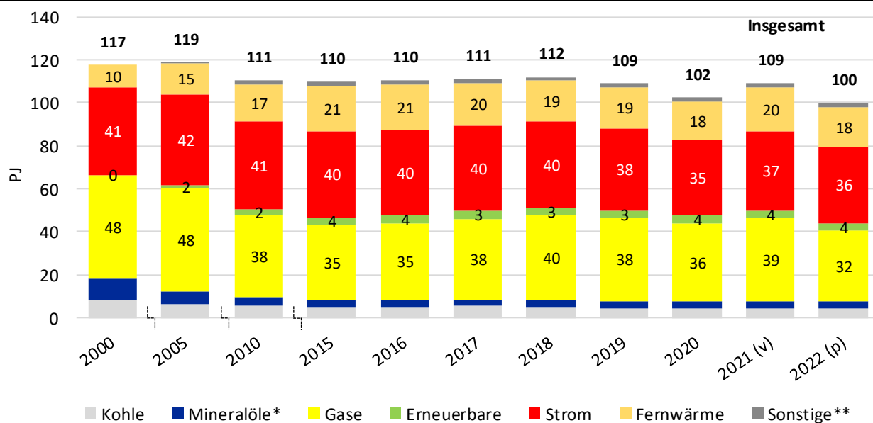
Abbildung 8: Entwicklung des Endenergieverbrauchs in der Industrie nach Energieträgern 2000-2022 (in PJ)
