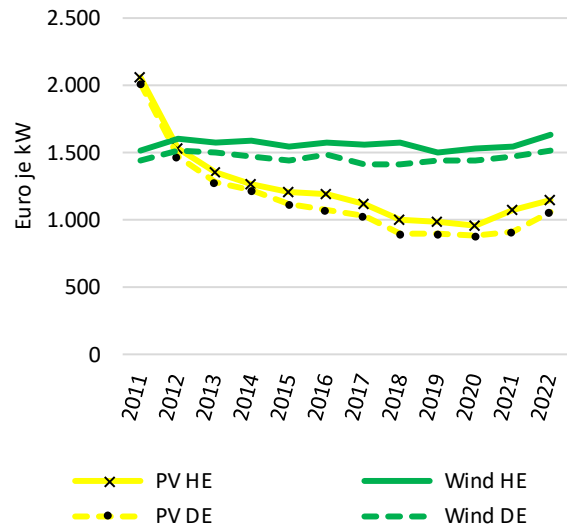
Abbildung 74: Entwicklung der spezifischen Investitionskosten für Photovoltaik- und Windenergieanlagen in Hessen und im Bundesdurchschnitt 2011-2022 (in Euro je kW installierter Leistung)
