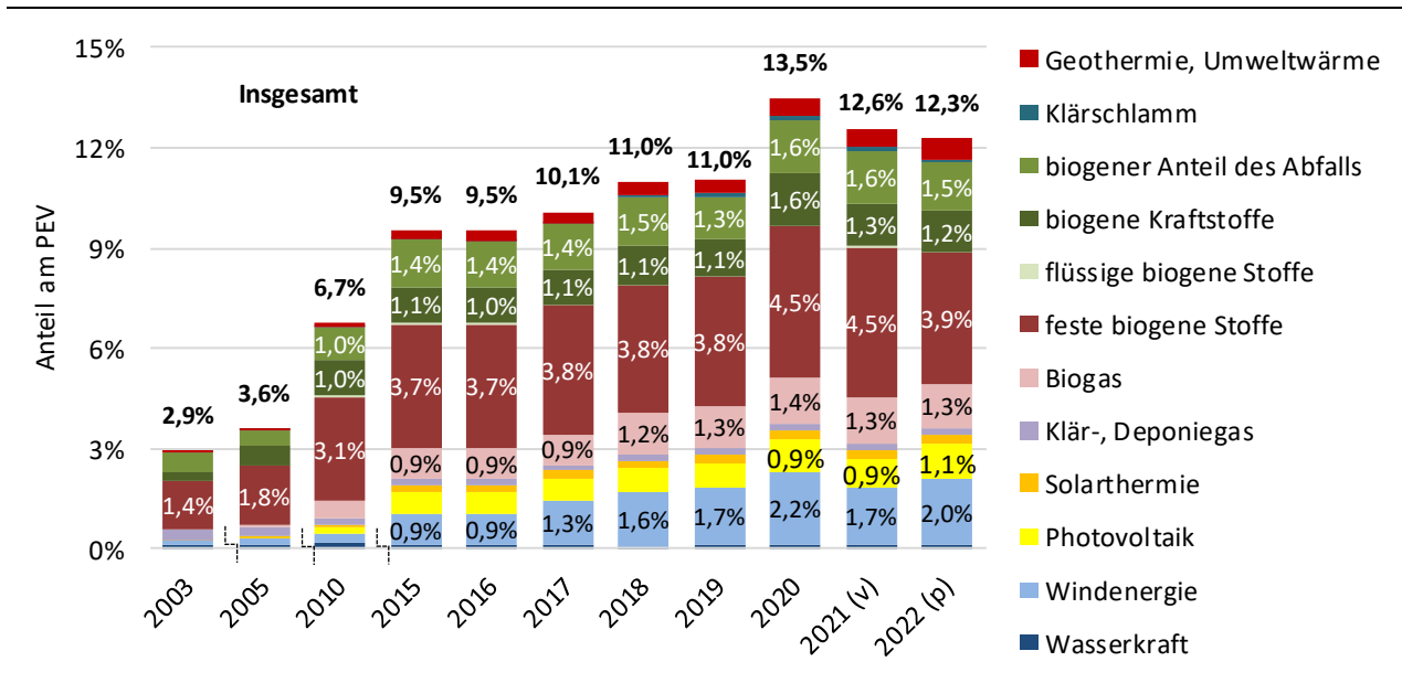
Abbildung 21: Anteile erneuerbarer Energieträger am Primärenergieverbrauch 2003*-2022 (in %)
