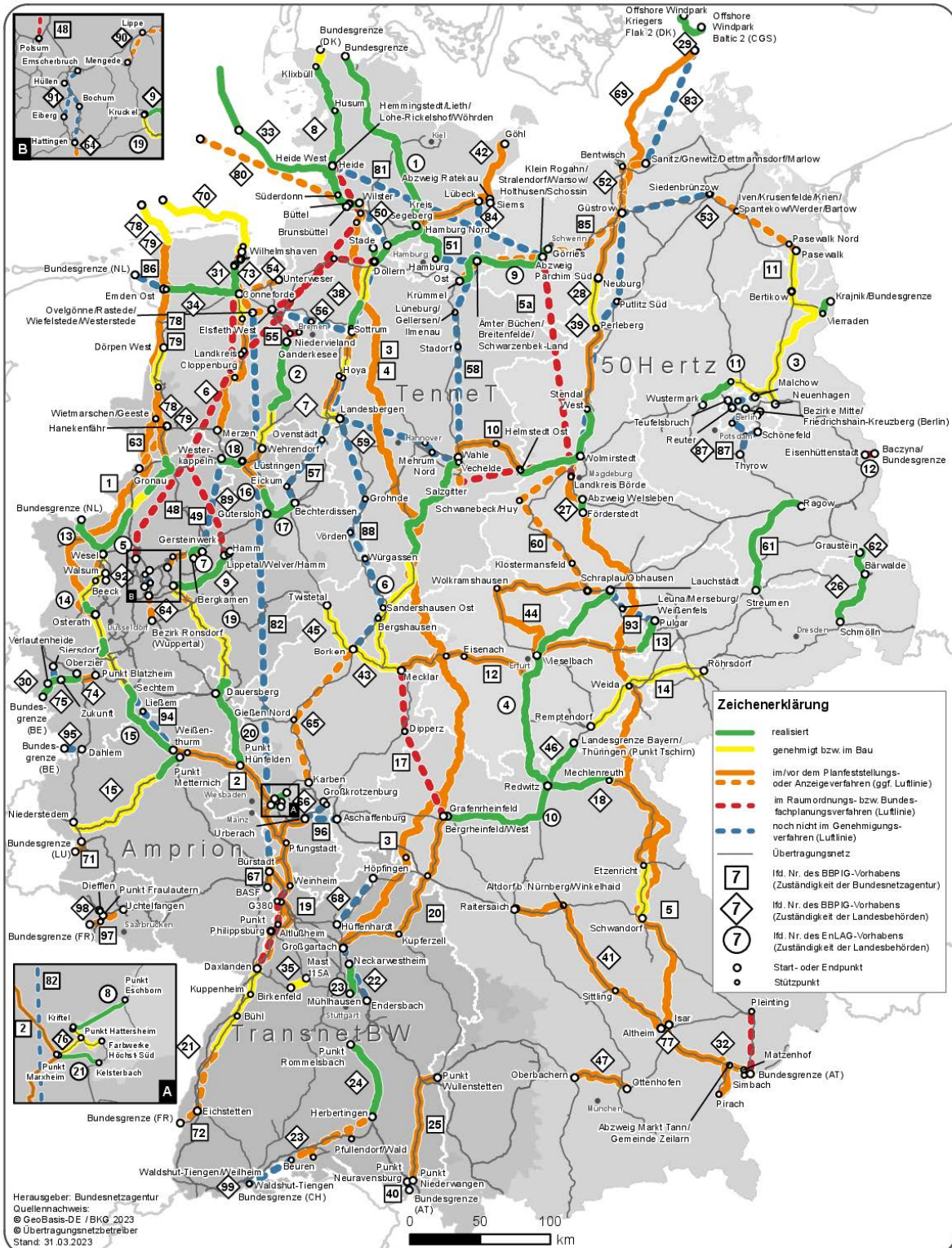
Abbildung 48: Stand der Vorhaben aus dem BBPIG und EnLAG zum 31.03.2023
