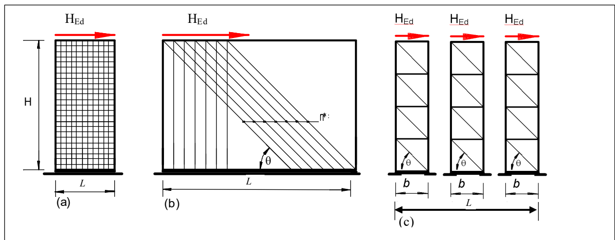
a) Rahmenmodell
