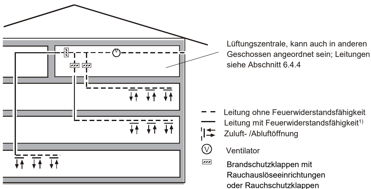
Bild 1.4: Lüftungsanlagen mit getrennten Hauptleitungen und gemeinsamer Außenluft- oder Fortluftleitung mit Rauchschutz
